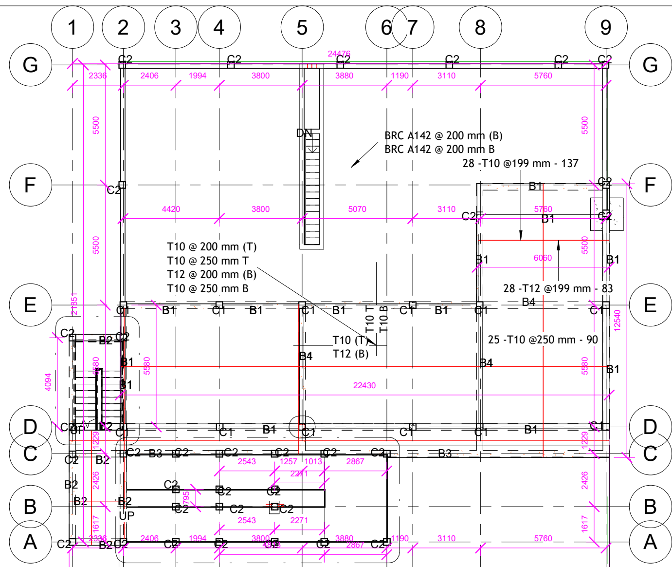
3 G.F Level 1 : 150
