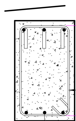
10 Beam B2 Section 1 : 10
