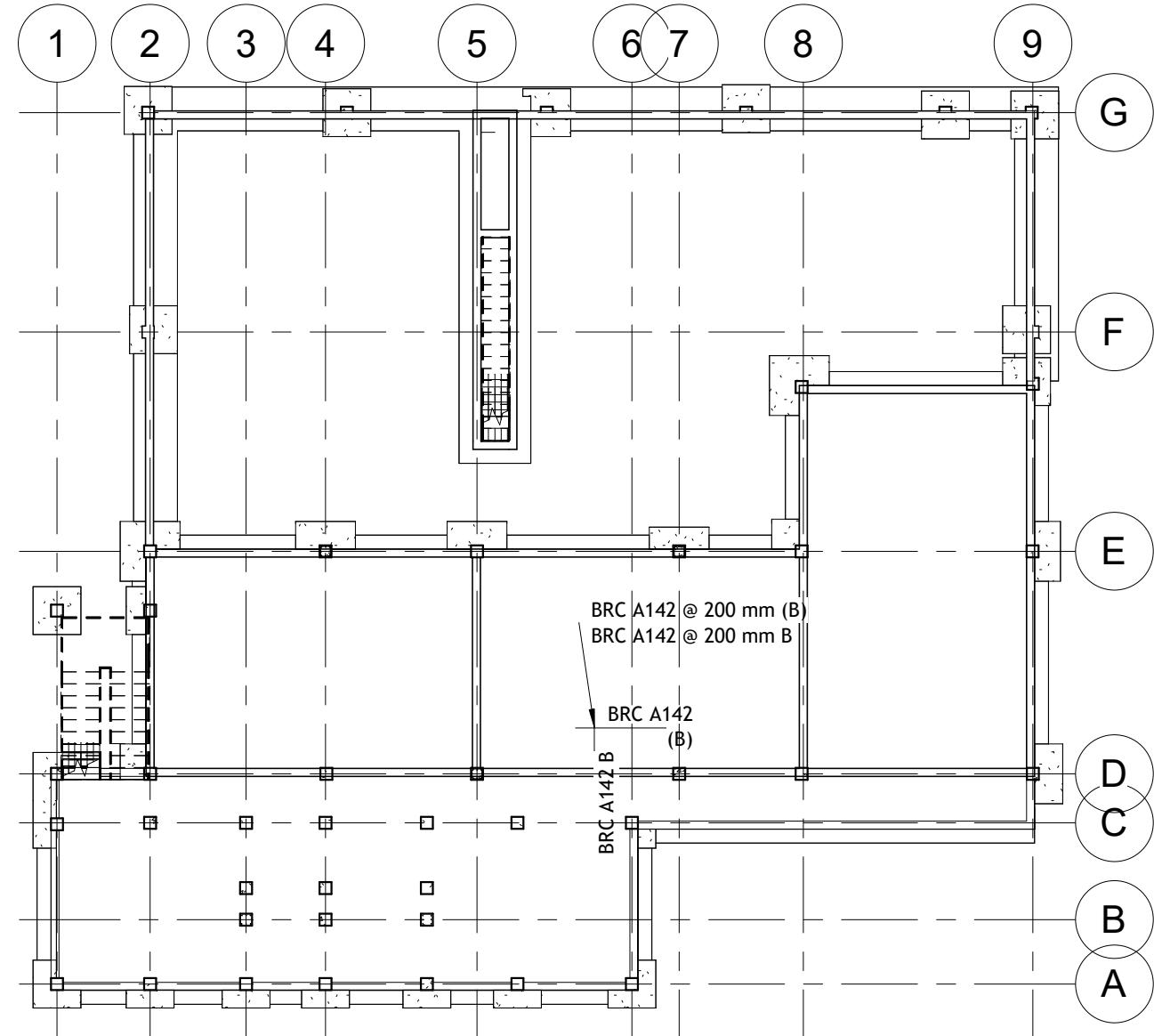
6 Basement 1 1 : 150
