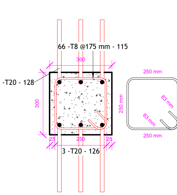
7 Column C1 1 : 10
