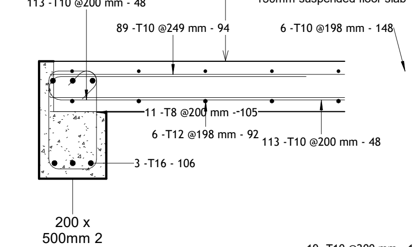
11 Beam B3 1 : 10
