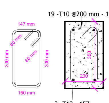
17 Beam B5 1 : 10
