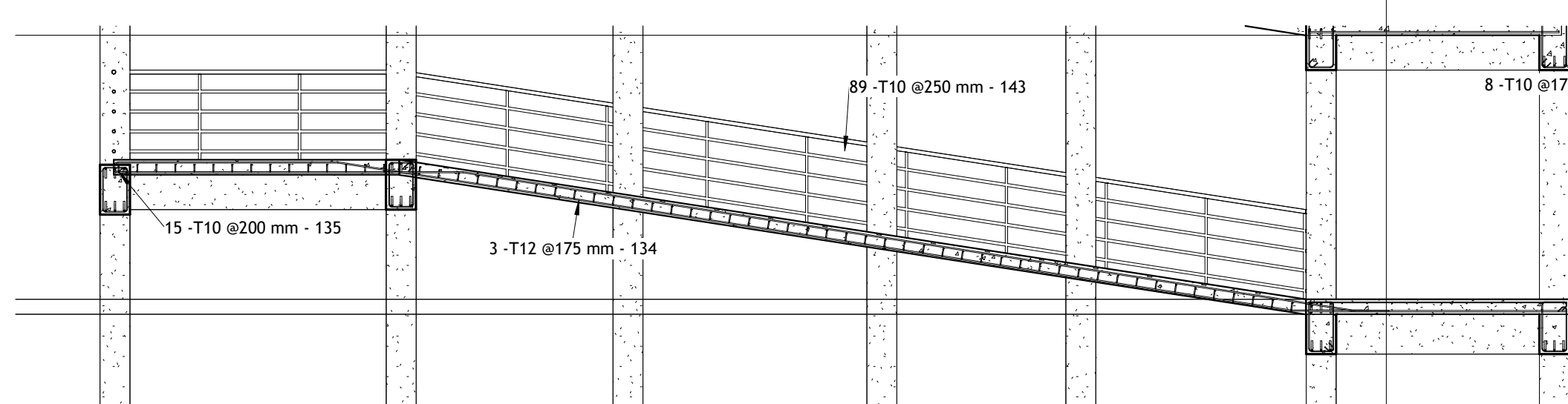
15 Ramp section 1 : 50
