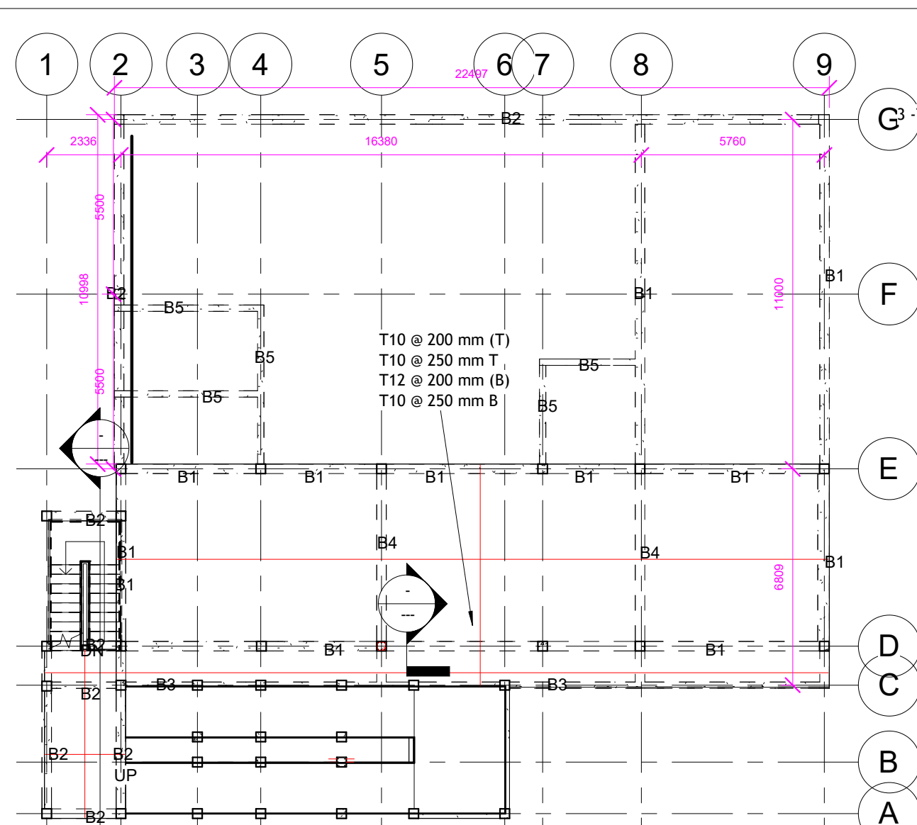
2 F.F Level 1 : 150
