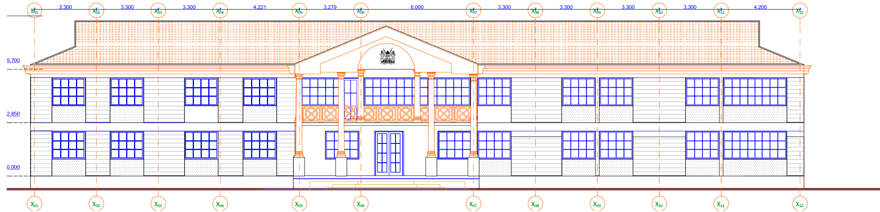
ELEVATION E 01
