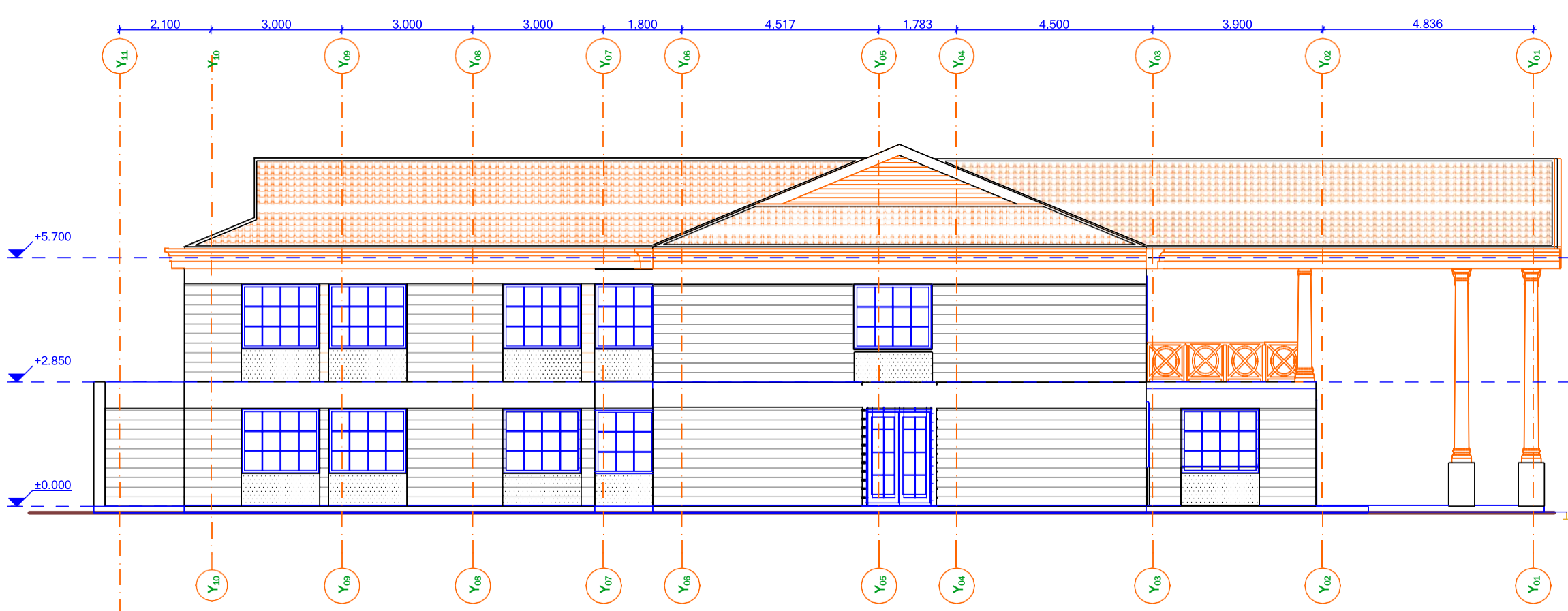
ELEVATION E 02
