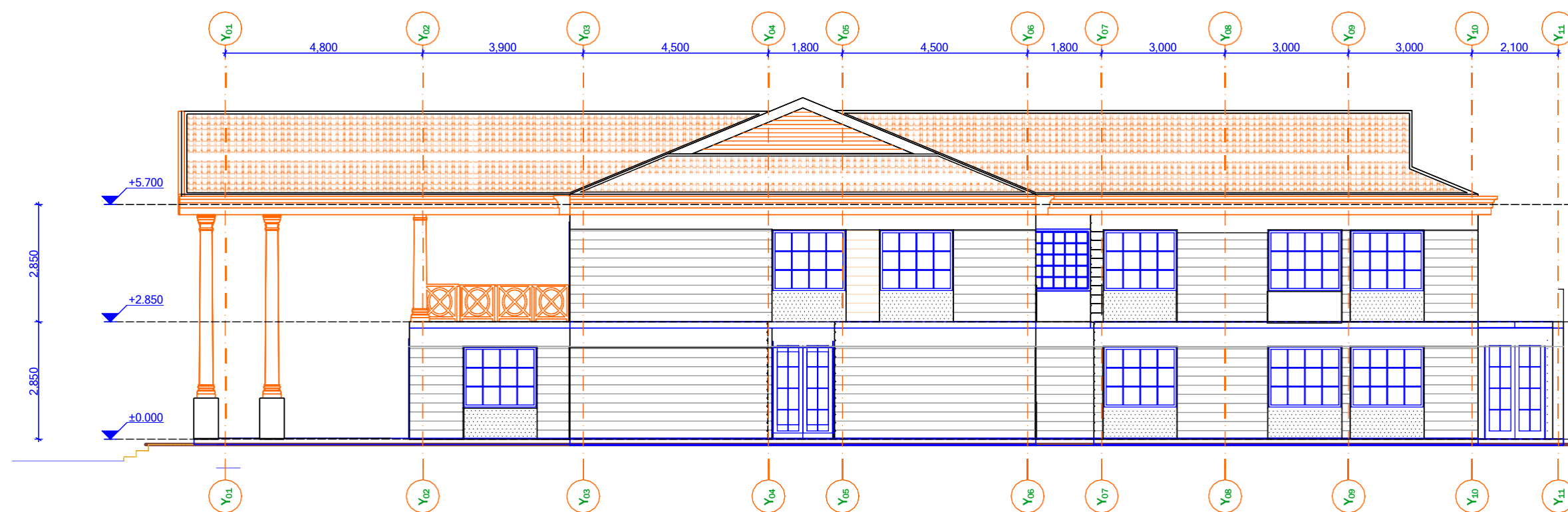
ELEVATION E 04
