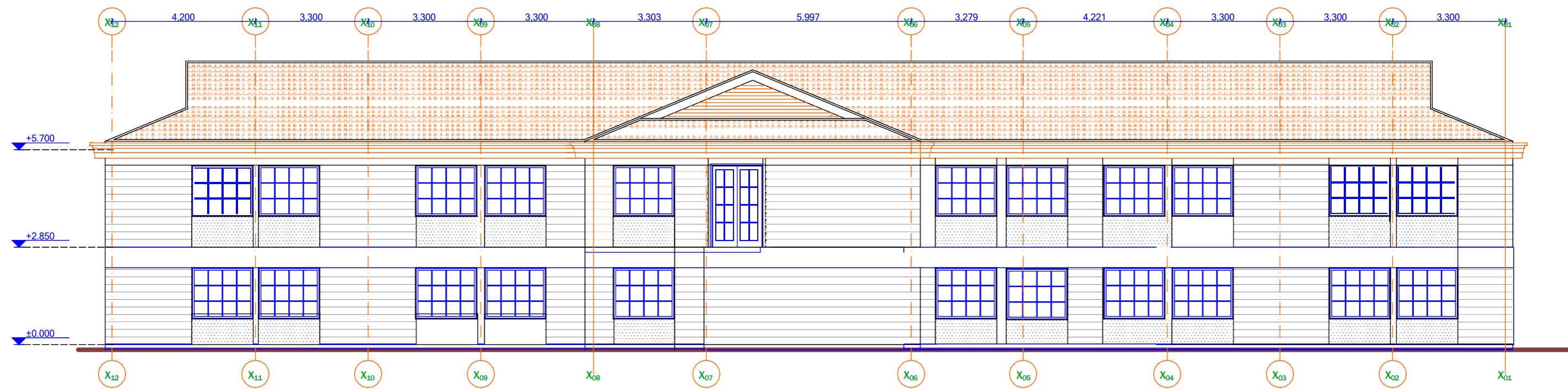
ELEVATION E 03
