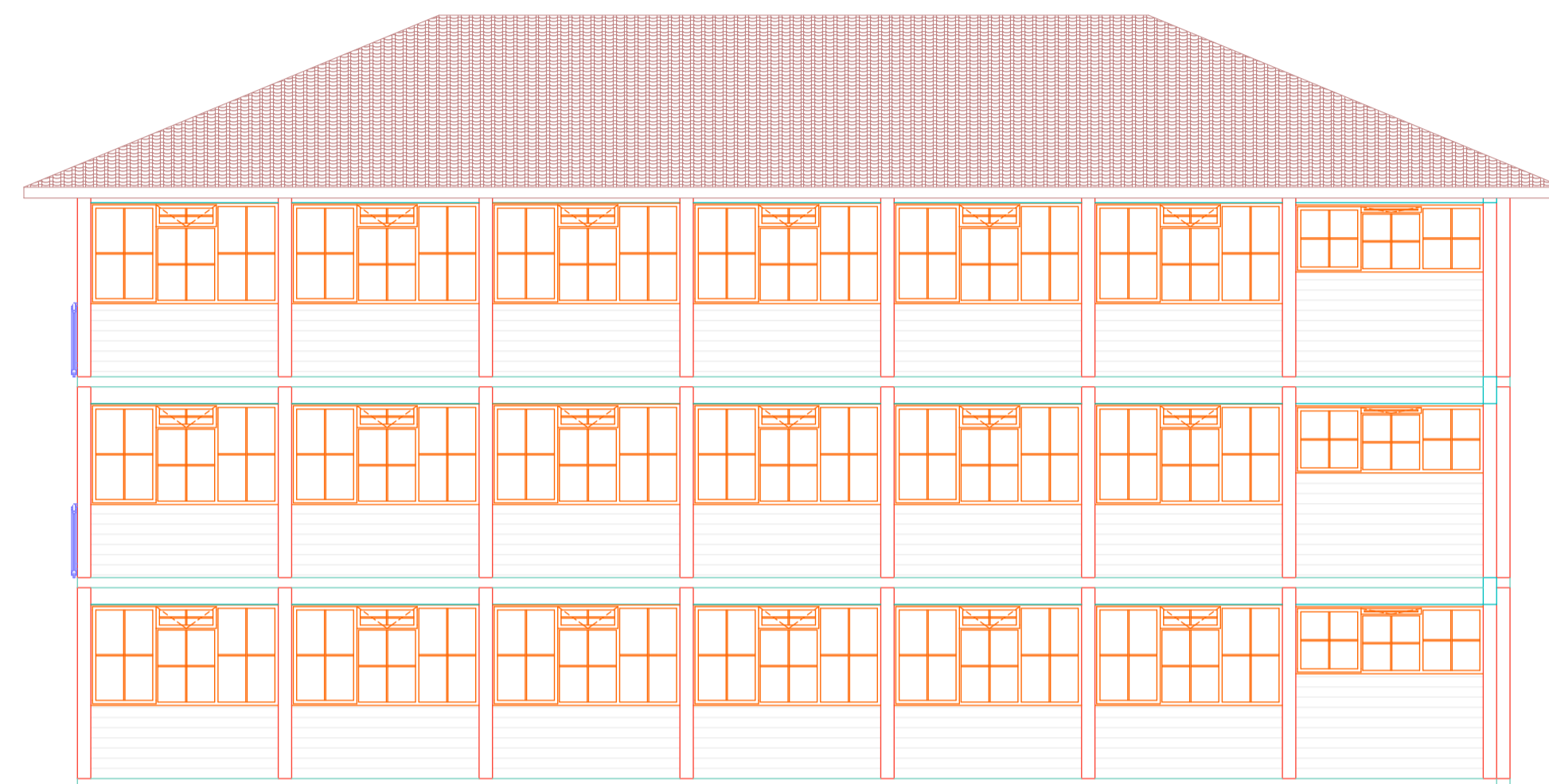
ELEVATION 04
