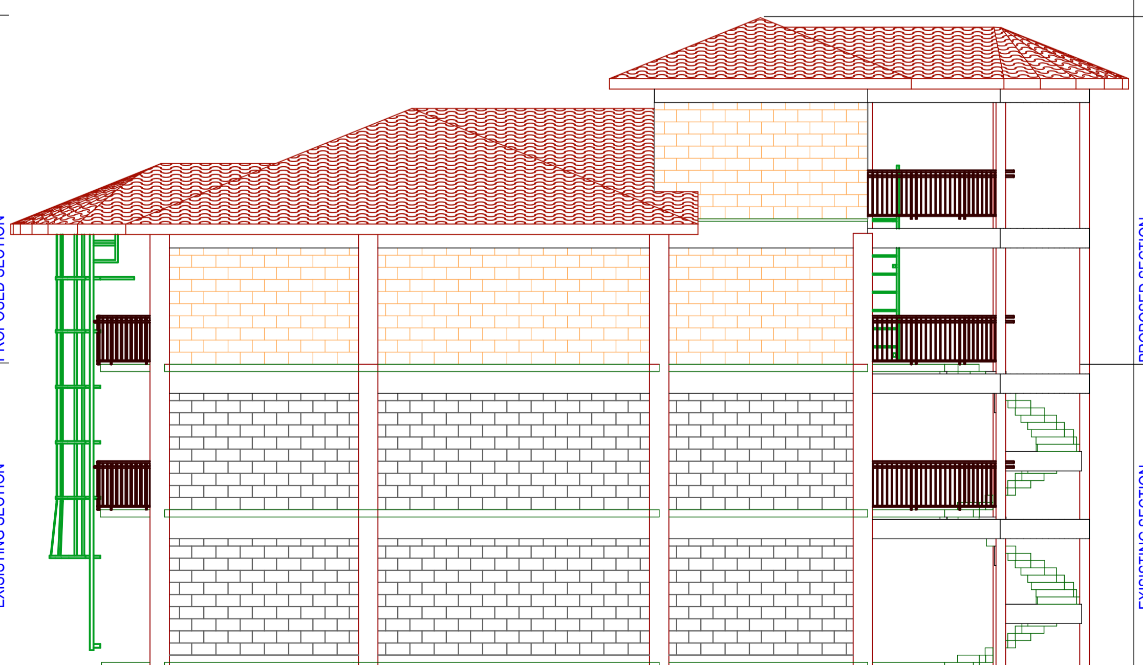
ELEVATION 04
