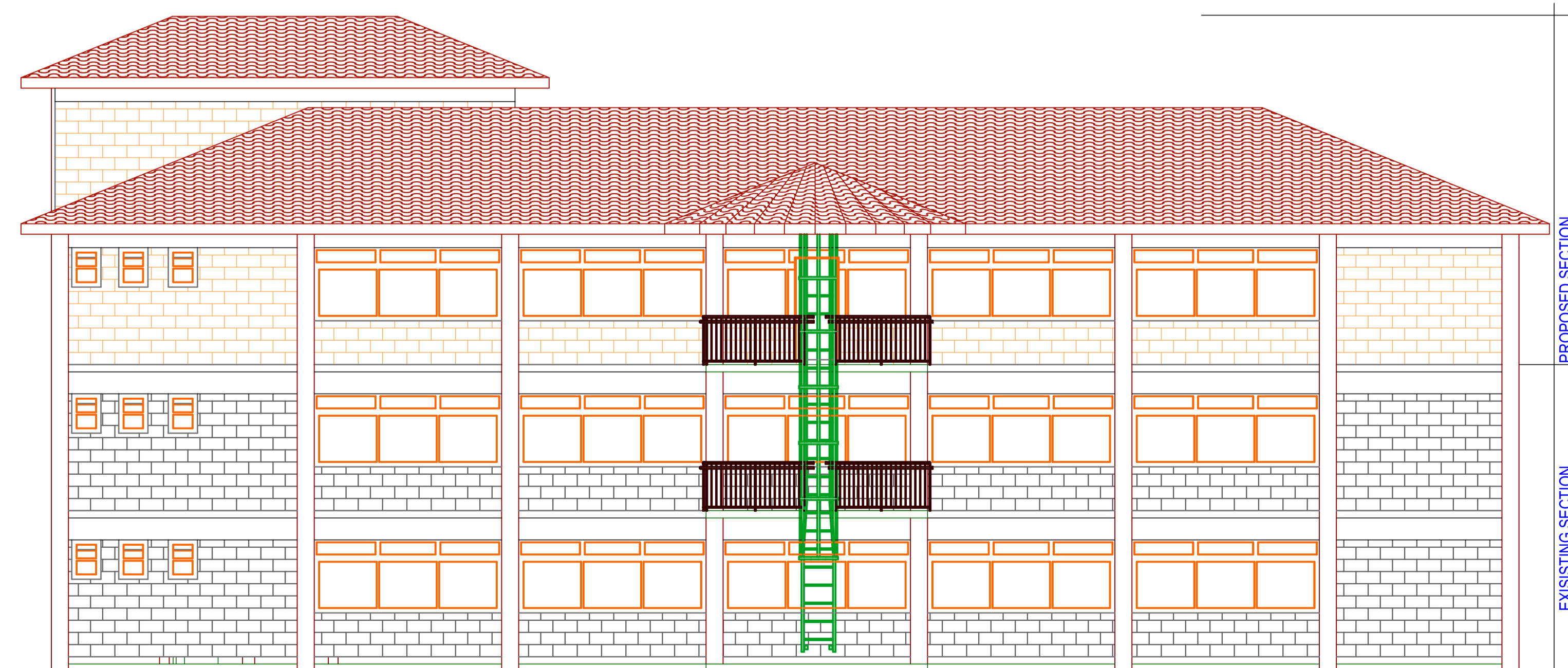
ELEVATION 02
