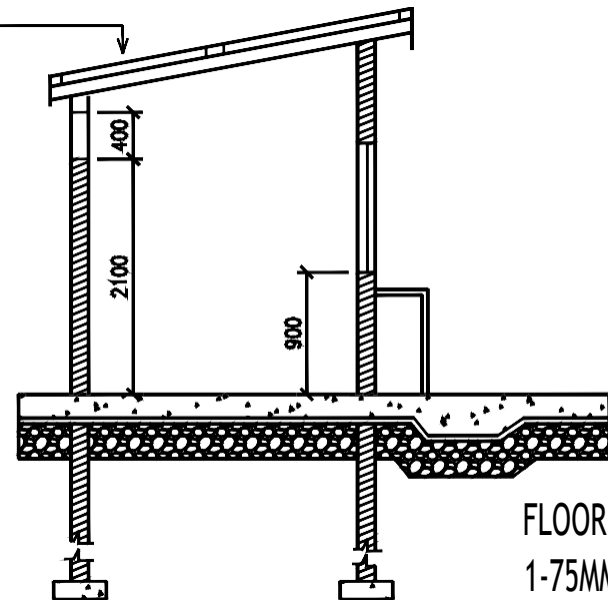
SECTION A5
