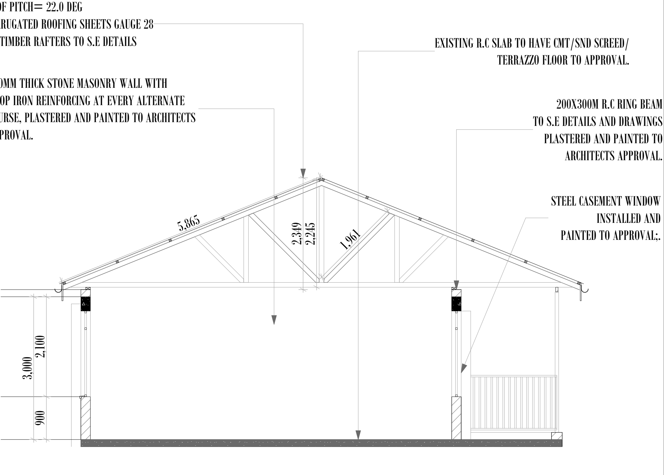
S-01 1:50
