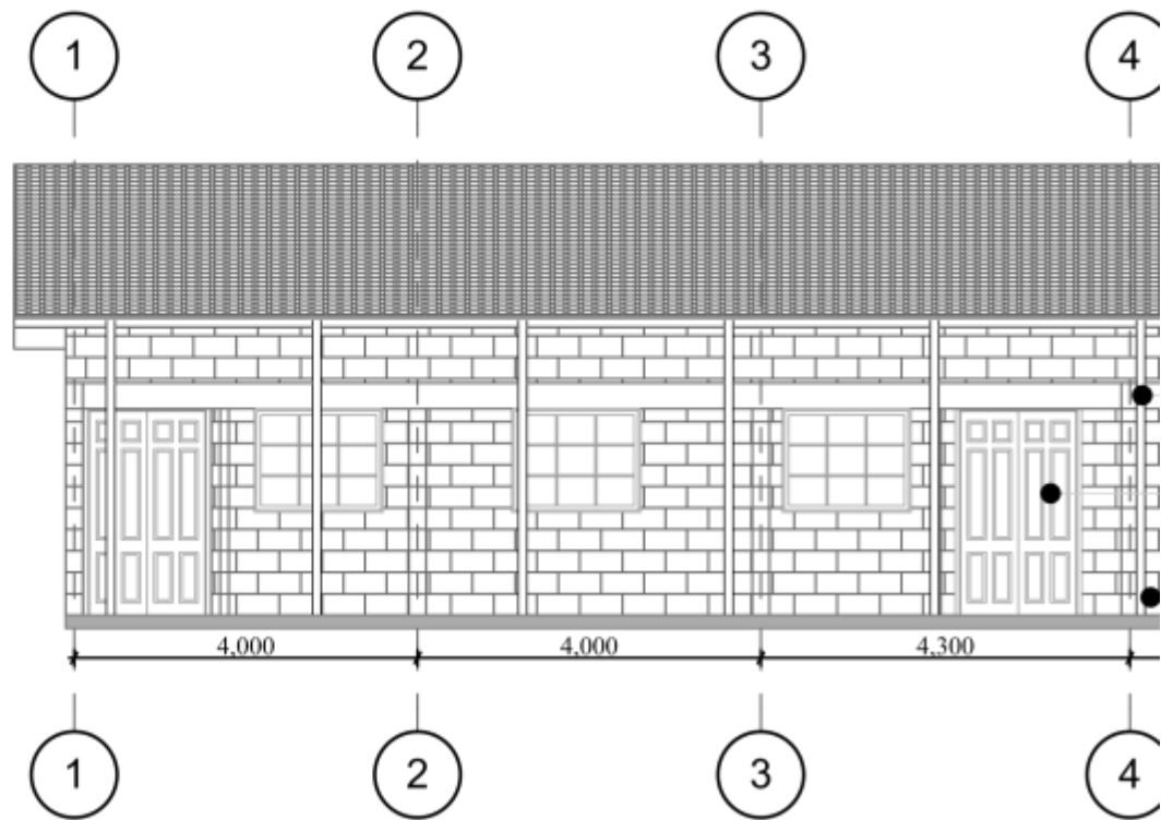
ELEVATION 03 1:100
