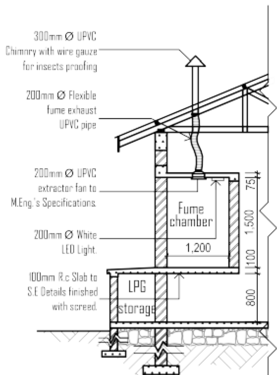
Section Y
