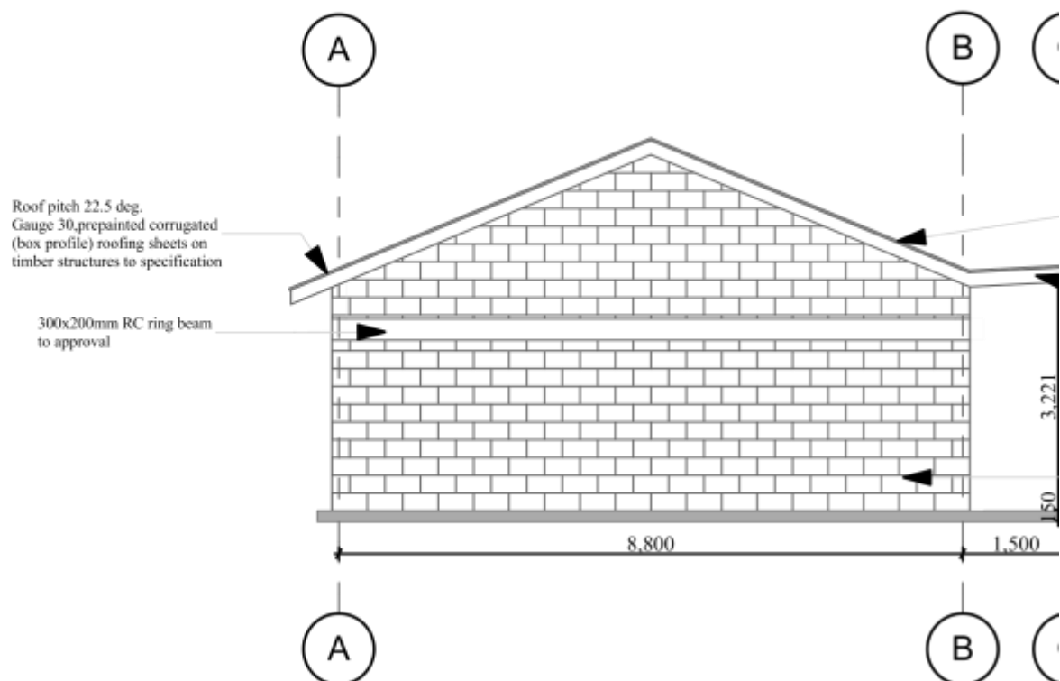
ELEVATION 04 1:100
